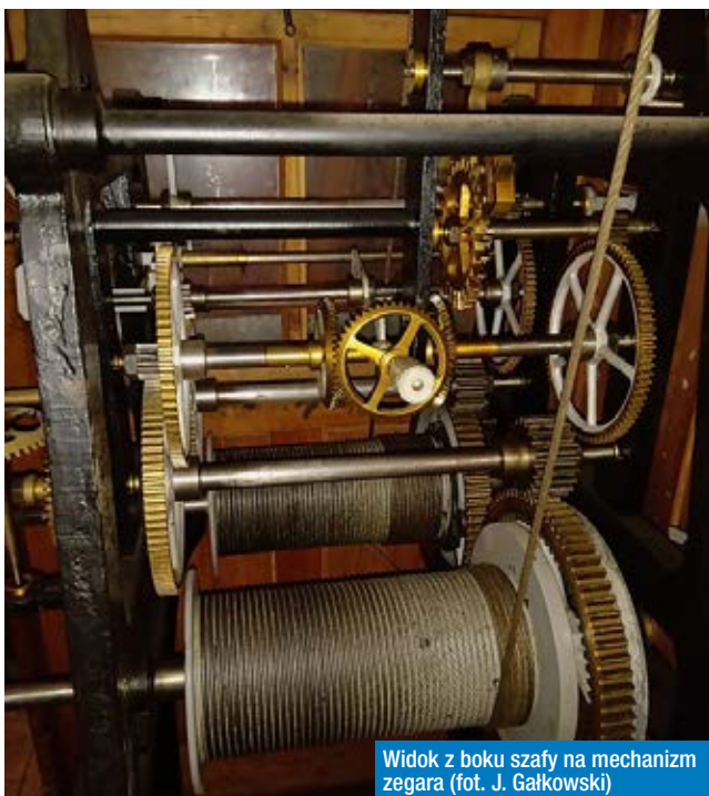
Widok z boku szafy na tylną część mechanizmu zegara (fot. J. Gałkowski)
